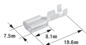
250型ファストンターミナル(コネクタ用)
