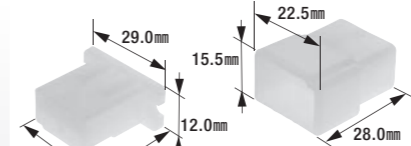
250型コネクタセット(4極)
