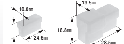
250型コネクタセット(2極)
