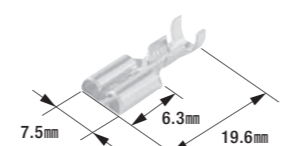
250型ファストンターミナル 24Kメッキ(コネクタ用)
