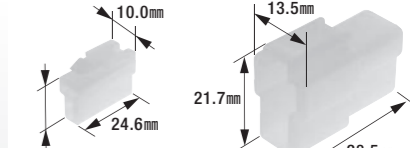
250型コネクタセット(2極ロック付)
