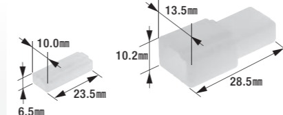
250型コネクタセット(1極)
