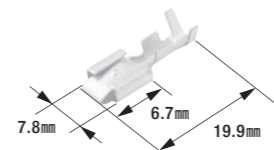
250型ファストンターミナル(1極コネクタ用)
