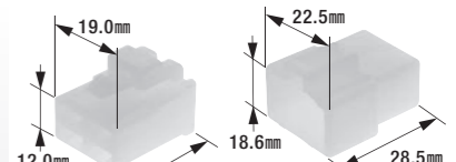
250型コネクタセット(4極ロック付)
