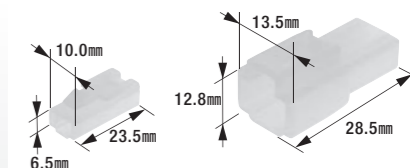
250型コネクタセット(1極ロック付)
