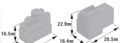
250型コネクタセット(3極ロック付)
