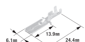
250型ファストンターミナル 24Kメッキ(コネクタ用)
