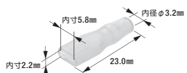
絶縁スリーブ(187型用)
