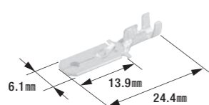
250型ファストンターミナル(コネクタ用)
