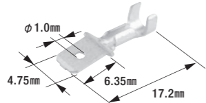
187型ファストンターミナル
